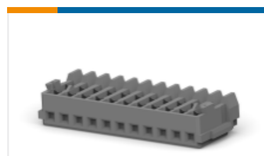
TE 零件编号 1-353293-1 MINI CT MT REC ASSY 11P GRAY
